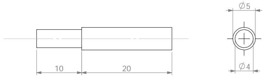
Axe de came
