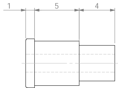
Glissière
