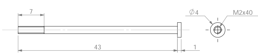
Tige de commande
