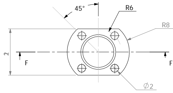
Bloc echappement
